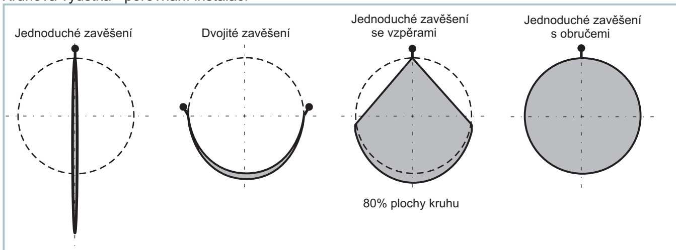
Kruhová vyústka - porovnání instalací
