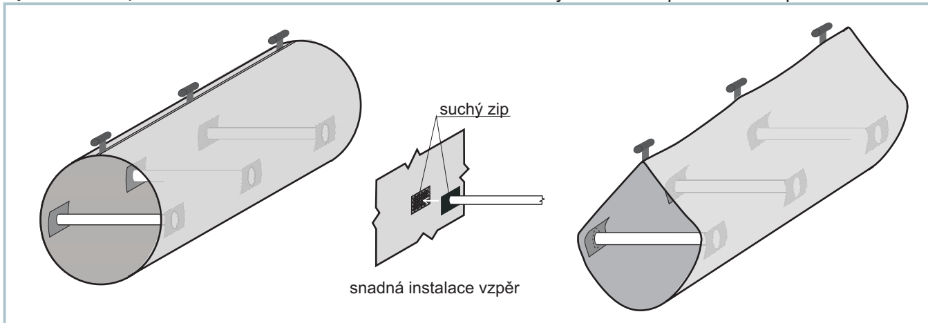
Vyústka se vzpěrami - nafouknutá
